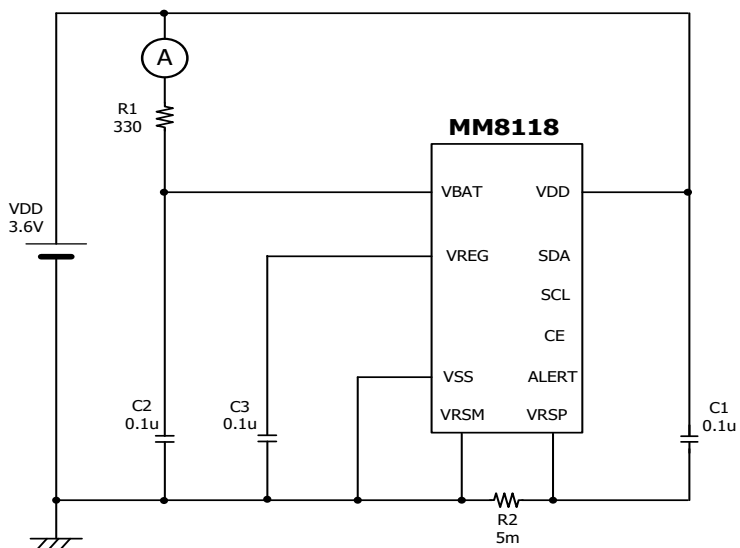
T5 : Pcell
