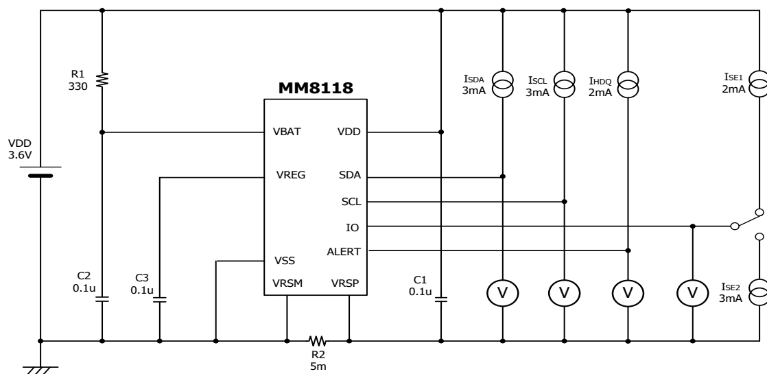
T6 : Vol,Voh
