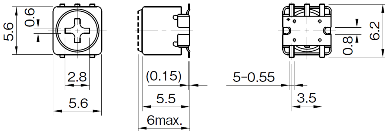
外形図
