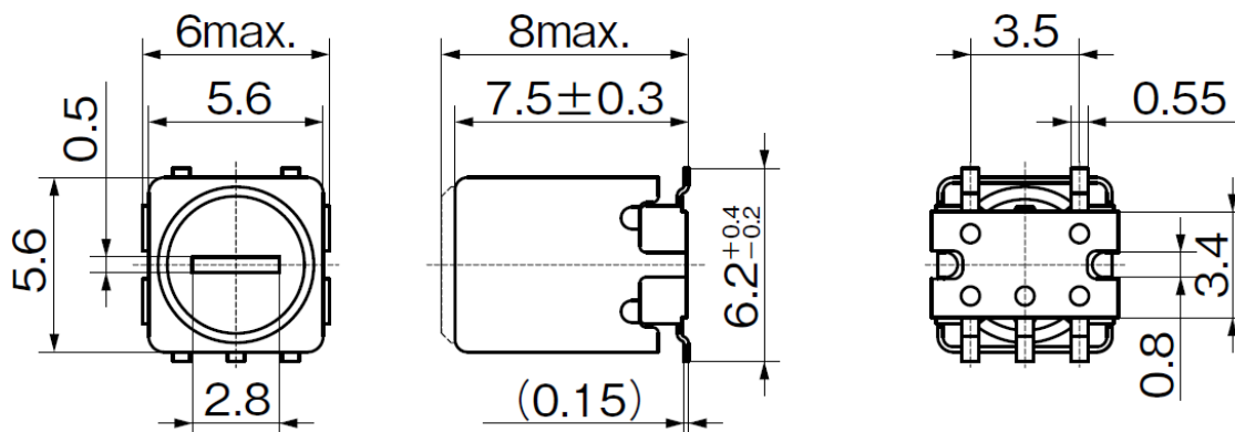
外形図
