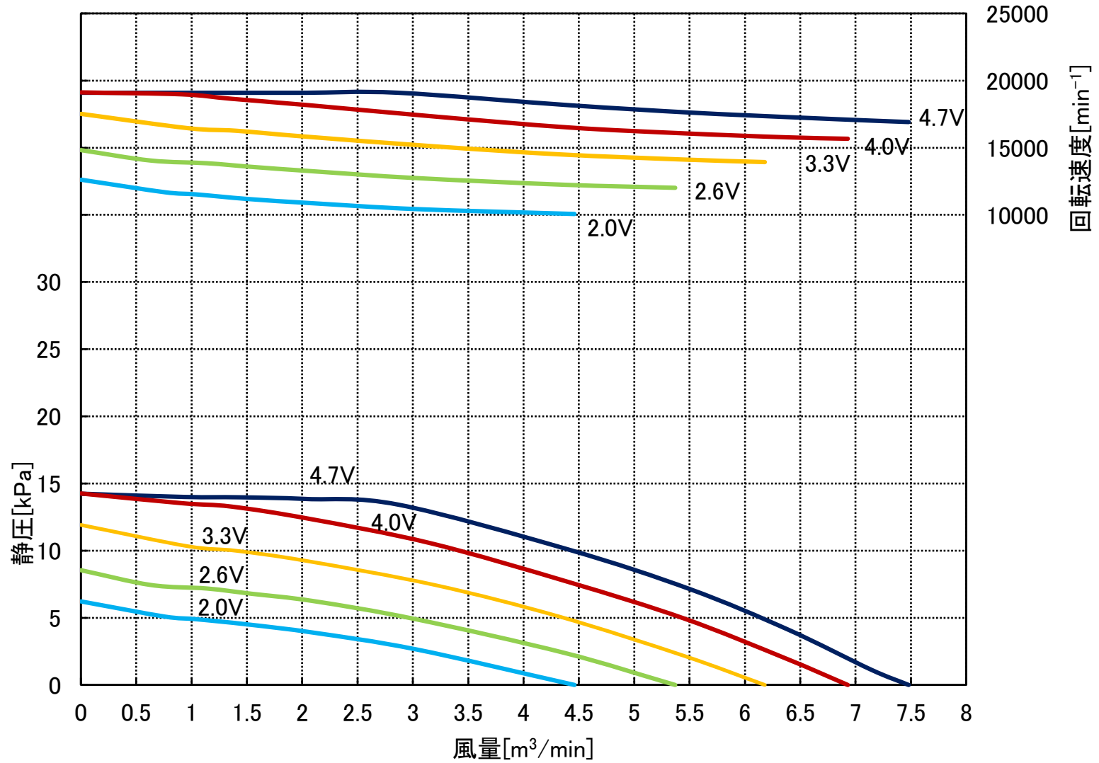
[参考値] 風量－静圧特性 70DCF-374 コントロール電圧別
