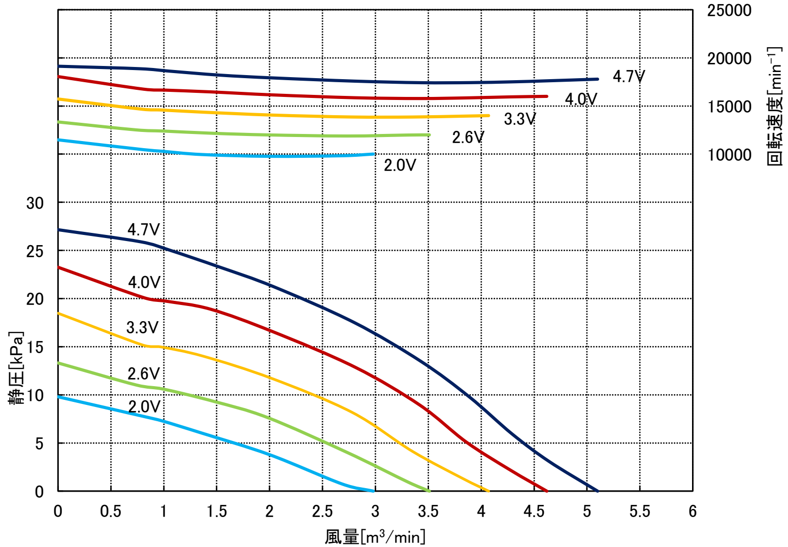
[参考値] 風量-静圧特性 70DCF-373 コントロール電圧別
