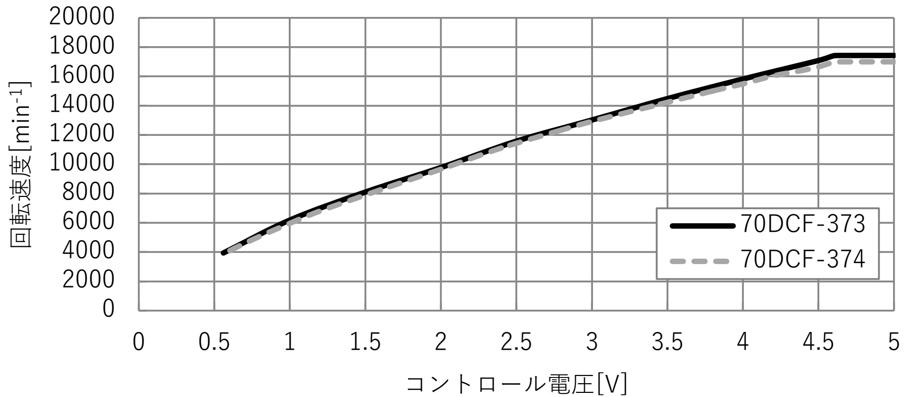
[参考値]コントロール電圧に対する回転速度（全開状態）
