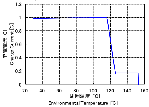
チップ温度制御・サーマルシャットダウン Chip Temperature Control · Thermal Shutdown
