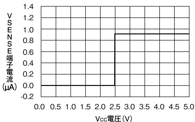
■ V_{SENSE} 端子電流— V_{CC} 電圧特性 (BAT=4.0V, 充電OFF)
