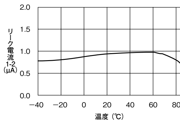
■ リーク電流1-2
