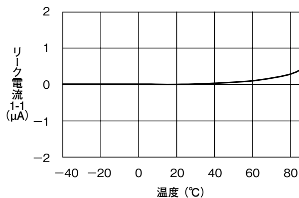
■ リーク電流1-1
