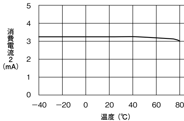
■ 消費電流2
