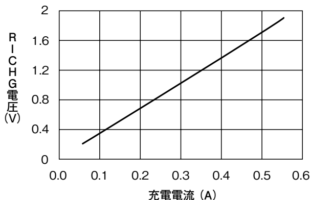
■ RICHG電圧—充電電流
