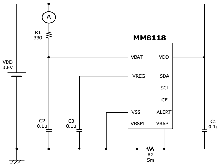
T5 : Pcell
