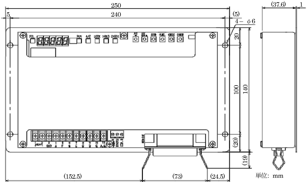
取付金具 (別売品) 取付寸法
